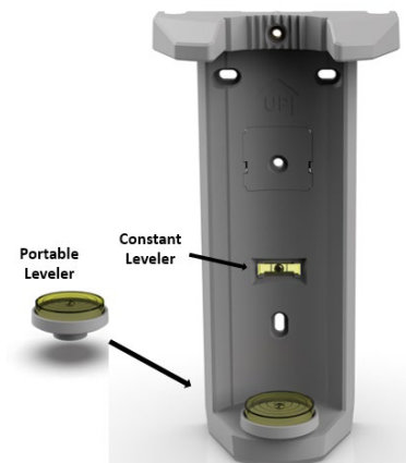
FIG. 1.2 – DETECTOR PARTS (CONT.)
